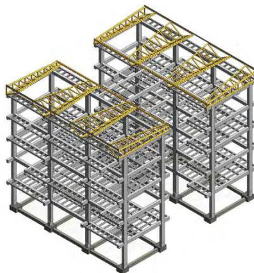
Sistema estructural aporticado en concreto con cimentación de zapata corrida y cubierta con cercas prefabricadas en guadua.
