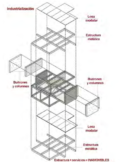
Estructura y los elementos de pisos, muros, buitrones para instalaciones y entresijos de la vivienda.
