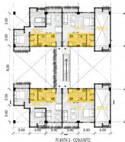
Plantas de pisos altos con distintos tipos de vivienda.
