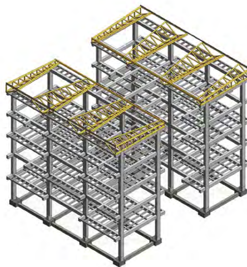
Sistema estructural aporticado en concreto con cimentación de zapata corrida y cubierta con cercas prefabricadas en guadua.
