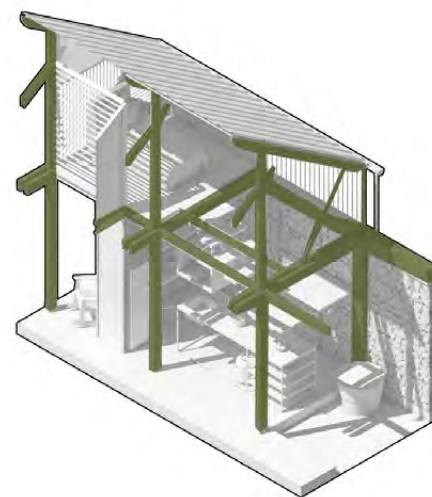
Sistema portante combinado: estructura principal en concreto complementada con madera.
