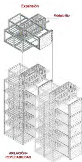
Ubicación alineada en altura del módulo fijo de servicios en la estructura del edificio.
